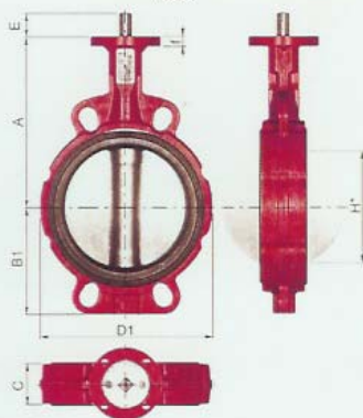
Typ D1 DN 25-700
