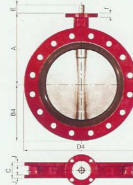
Typ D4 DN 150-1200
