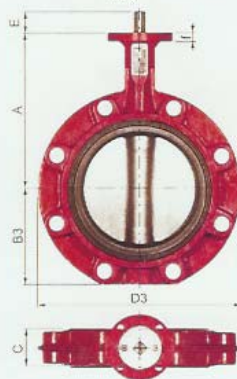
Typ D3 DN 50-400
